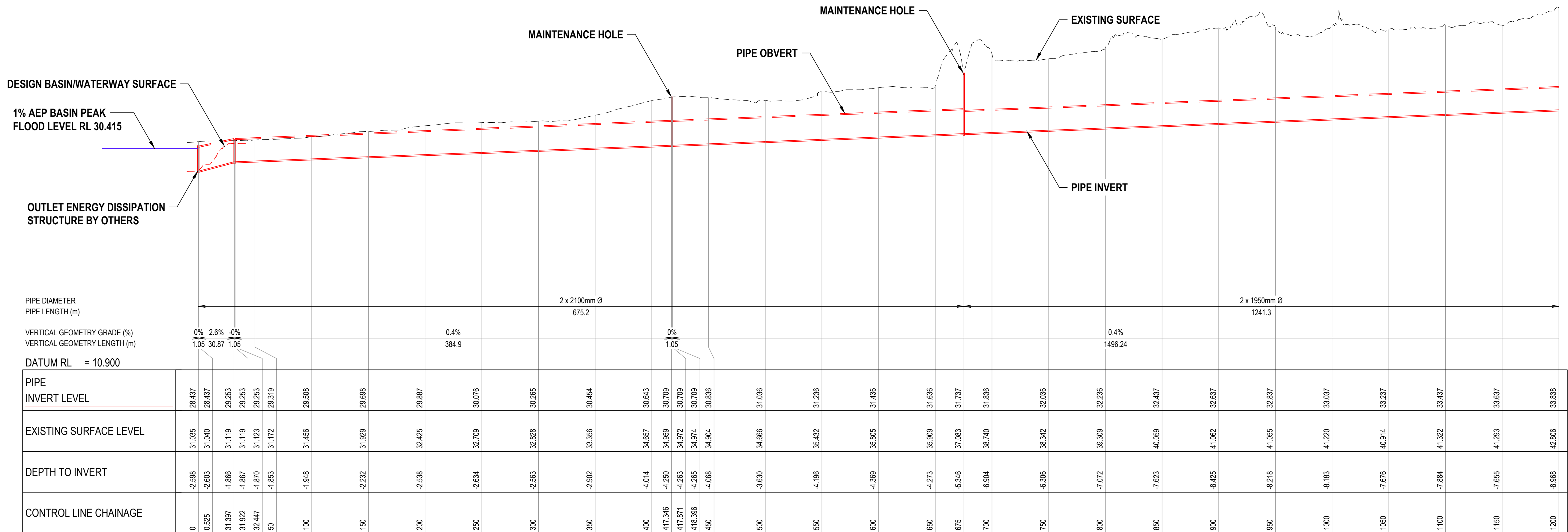
1% AEP DIVERSION PIPE LONGITUDINAL SECTION SCALE H 1:2000 V 1:200
